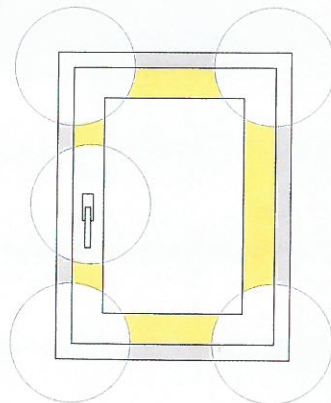
Fig. 2: punti di chiusura in una finestra dotata di accessori antieffrazione
